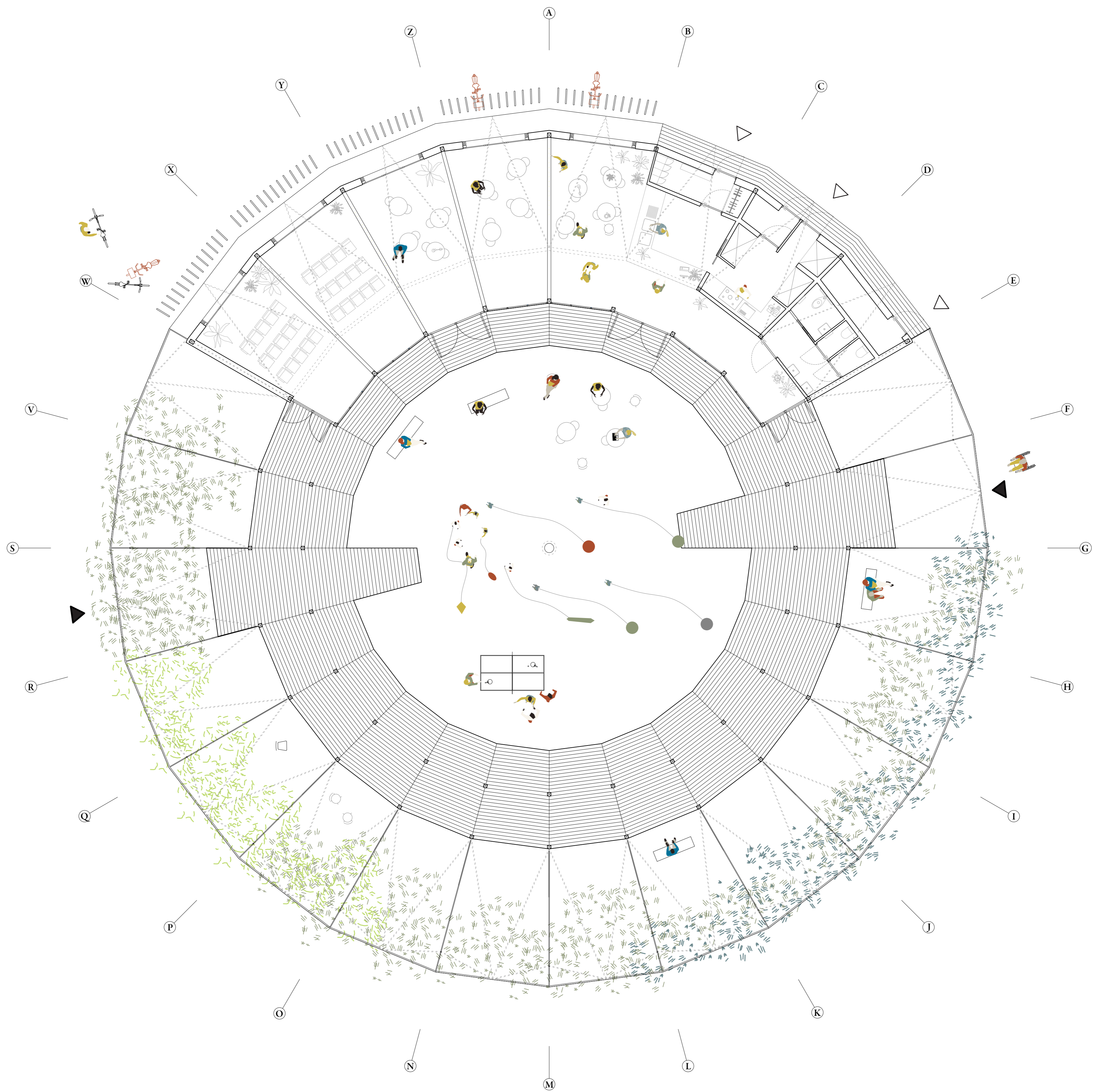
Pianta di progetto scala 1:100
