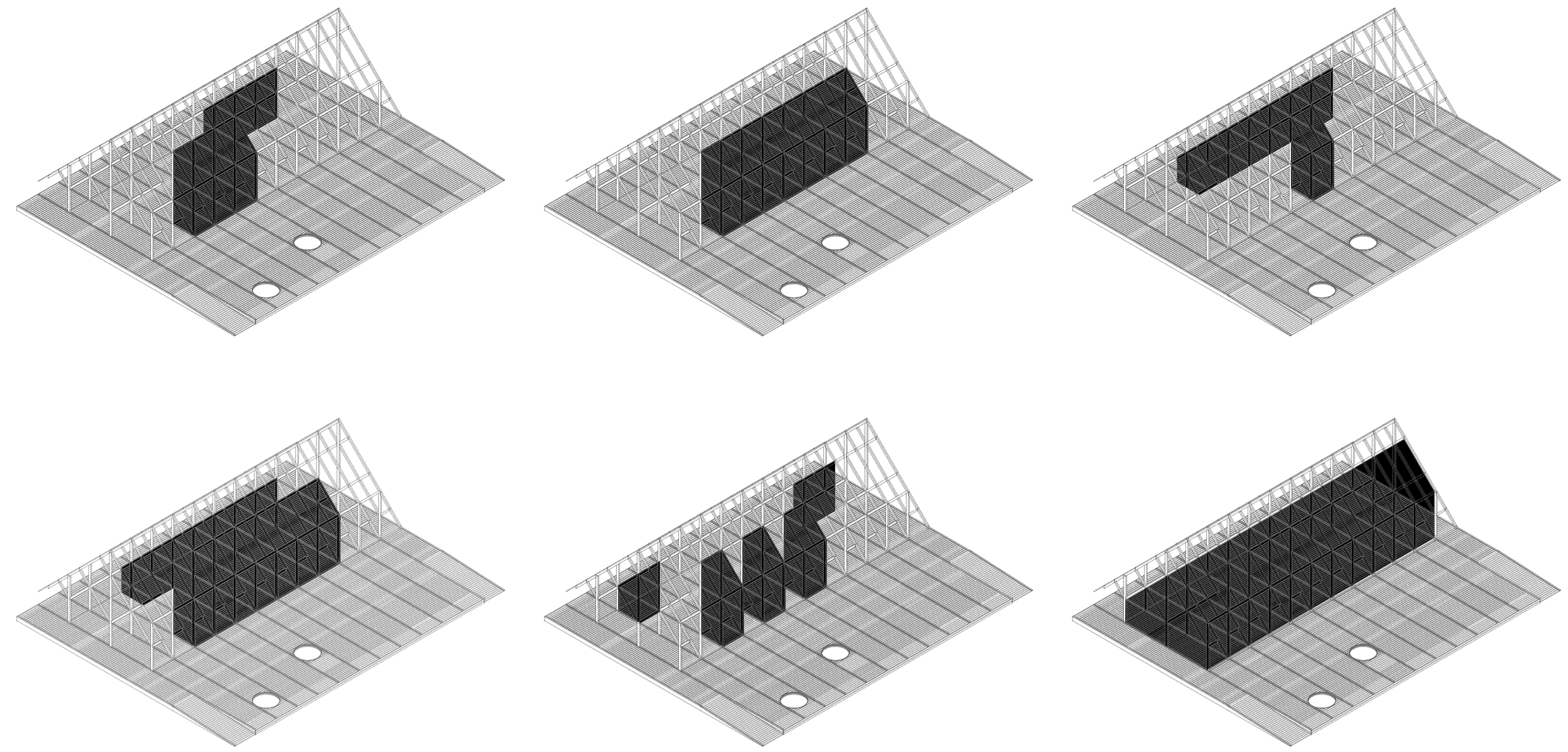
DIAGRAMMA: FLESSIBILITÀ DELLO SPAZIO
