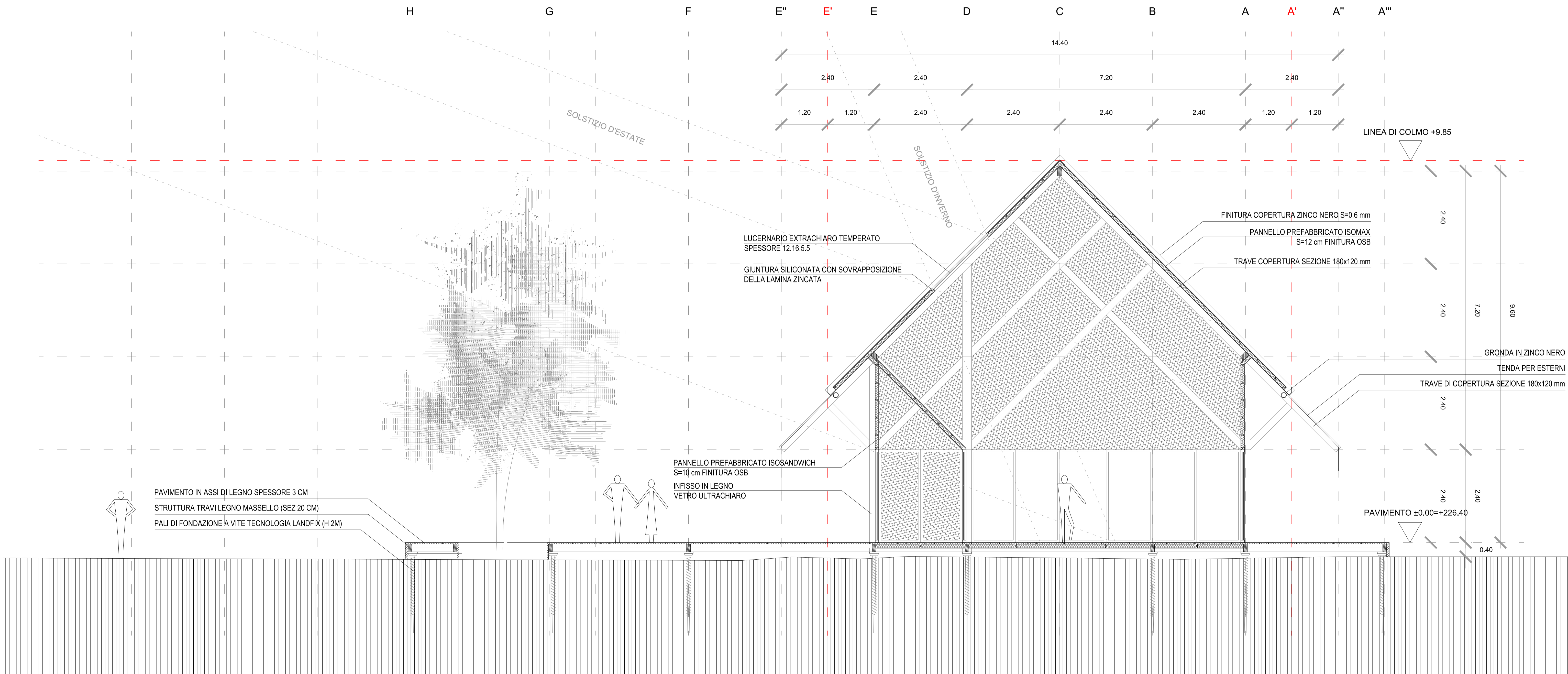
SEZIONE COSTRUTTIVA TRASVERSALE SCALA 1:50
