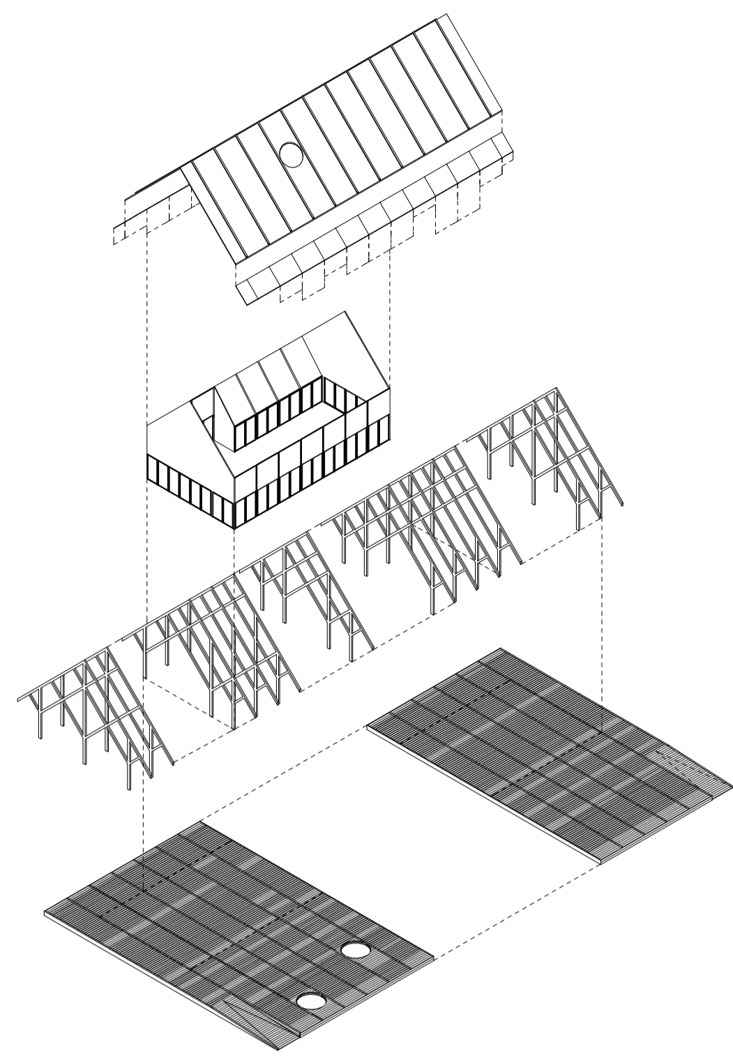
VISTA ASSONOMETRICA: ELEMENTI ARCHITETTONICI
