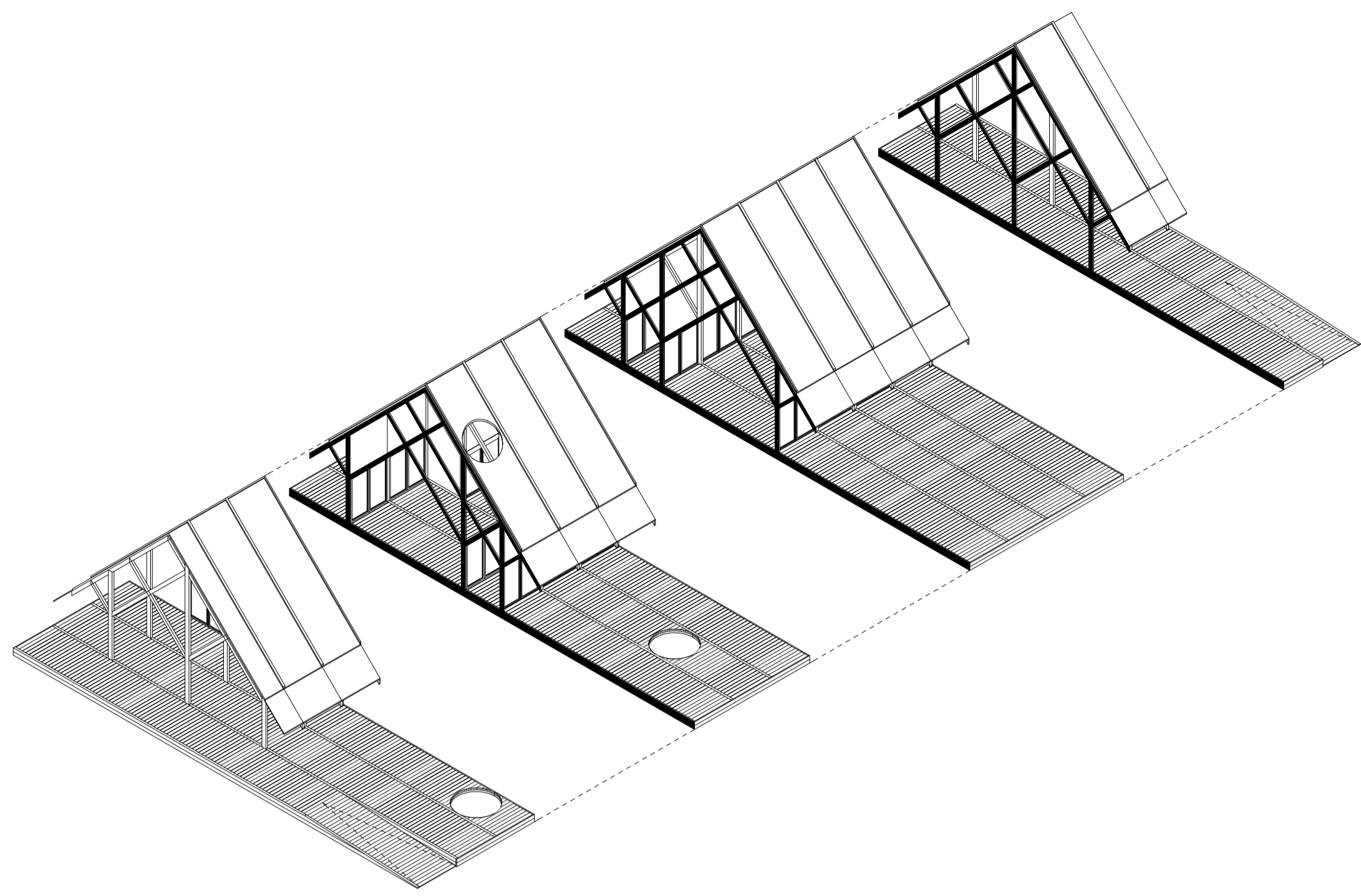
SEZIONE ASSONOMETRICA: CAMBIAMENTI STRUTTURALI E DIVERSE SPAZIALITÀ FUNZIONALI
